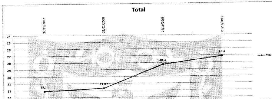
Figura 1. Comportamiento histórico de los niveles del pozo pz-19-0024.
